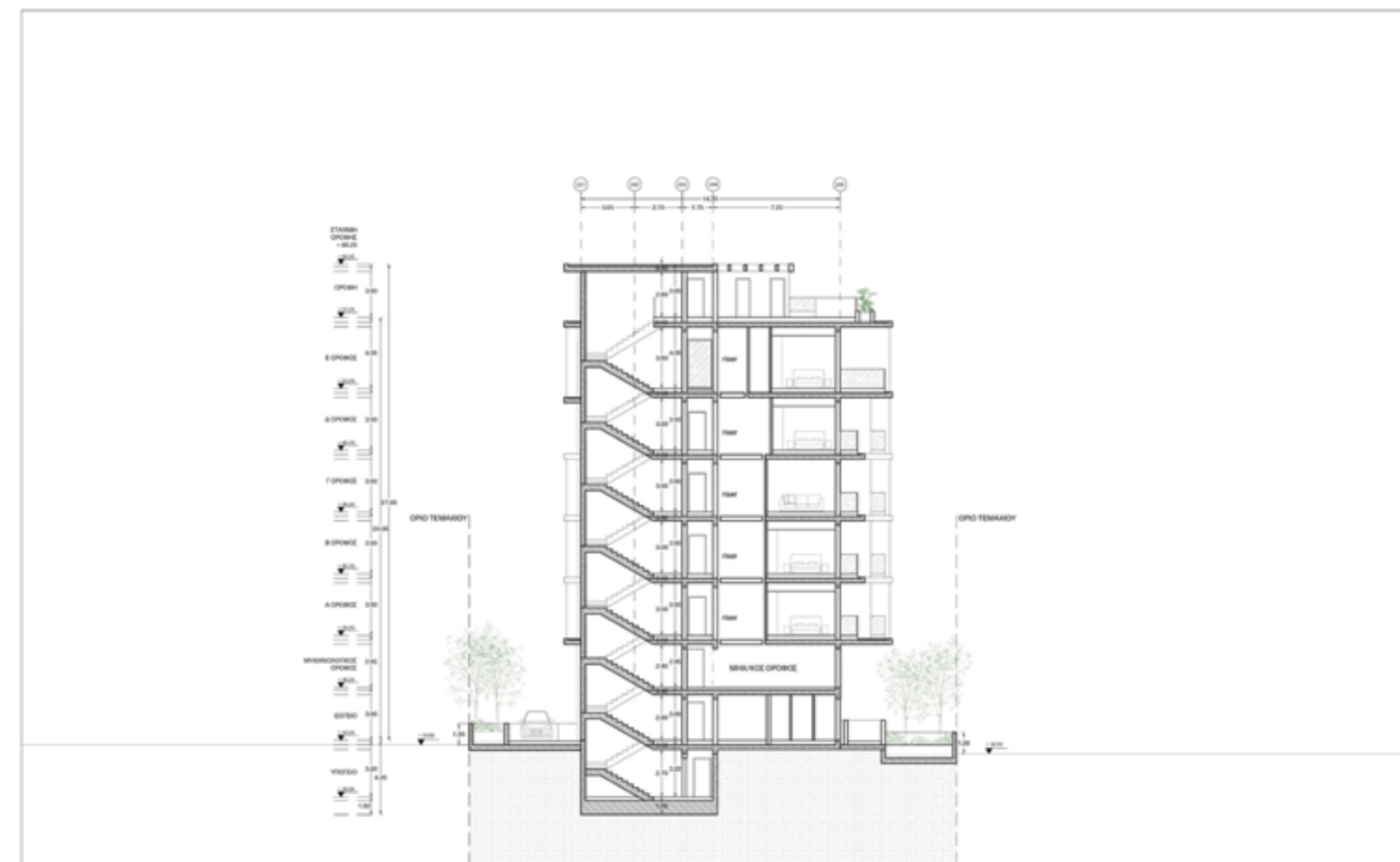
Section A-A
